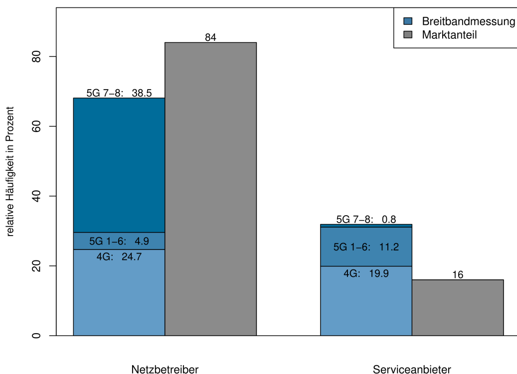
Abbildung 4.5: Mobile Breitbandanschlüsse: Verteilung der Messungen auf Netzbetreiber und Serviceanbieter im Vergleich zur Referenzverteilung. Für die Ergebnisse der Breitbandmessung mit blauem Hintergrund sind die Anteile für die drei Gruppen 4G-Messergebnisse über alle Bandbreitklassen, 5G-Messungen in den Bandbreitklassen 1 bis 6 und 5G-Messergebnisse in den Bandbreitklassen 7 und 8 farblich voneinander abgehoben (Quelle Referenzverteilung: Bundesnetzagentur, Stand: 17.12.2025, Zeitraum 30.06.2025).
