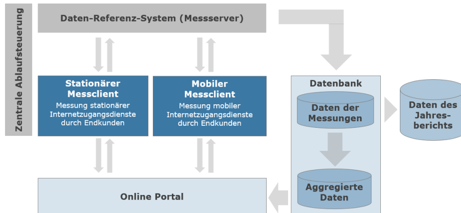
Abbildung 2.1: Übersicht Messkonzept.
